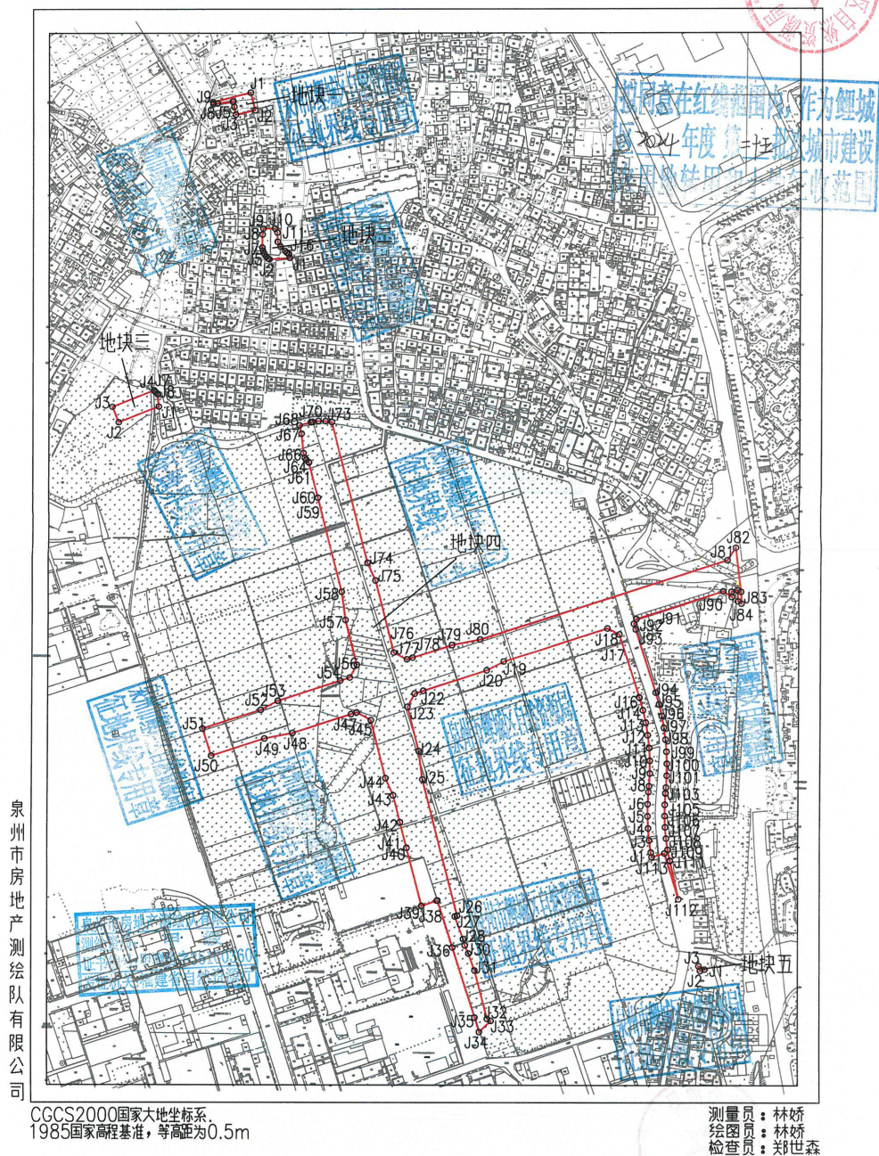
城中村改造配套道路工程（江南新区综合配套项目浮桥一期）（农转部分）勘测定界图
